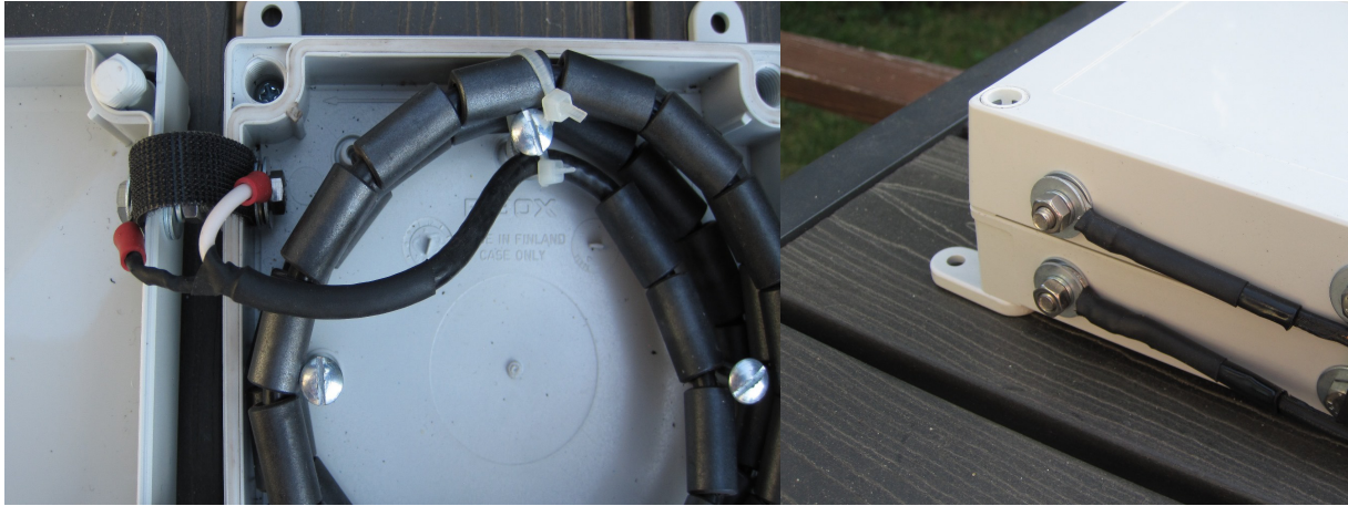
Détails des connexions de sortie, dans et hors de la boîte.
